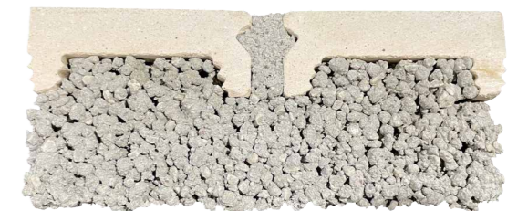
Beispiel Verlegung auf Drainagemörtel – Bettung und Fixierung ohne Haftschlämme
